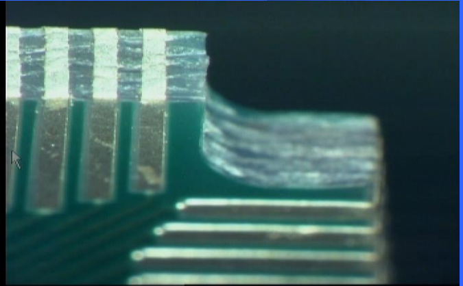
側面・凹凸面への配線パターン
